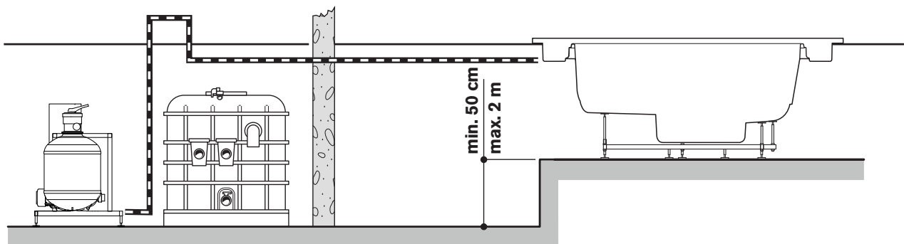
Spa Pack + Standardowym zbiornikiem kompensacyjnym
