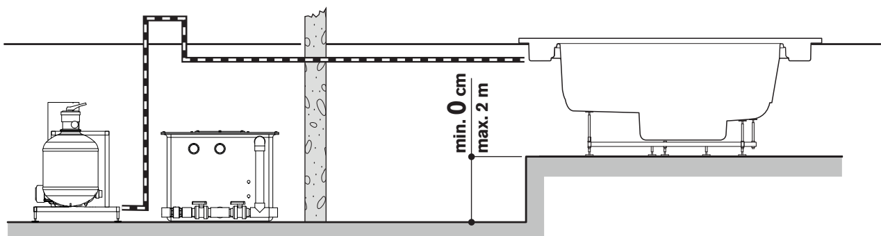
Spa Pack + Niskim zbiornikiem kompensacyjnym
